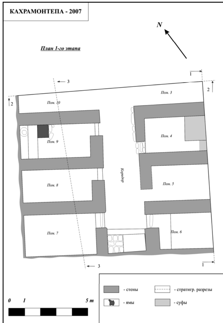
Рис. 2. План Кахрамонтепа 1 этажа.
